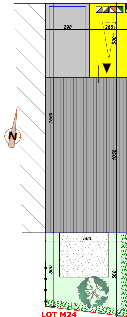
PLAN MASSE - Ech: 1/150
